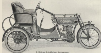
2. Kleiner dreirädriger Motorwagen. Übergangstyp vom Motorrad zum Motorwagen.
